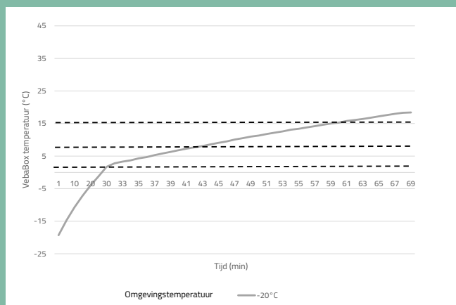
Verwarmingsprestatie bij omgevingstemperatuur Model B Cool
