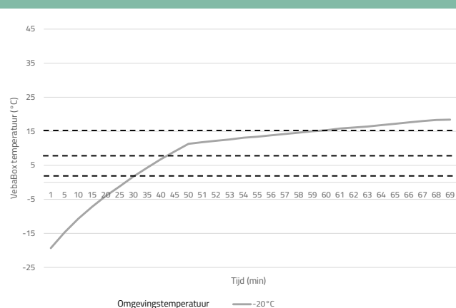
Verwarmingsprestatie bij omgevingstemperatuur Model I Cool
