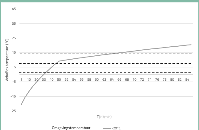
Verwarmingsprestatie bij omgevingstemperatuur Model O Cool
